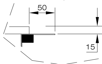
optional Fliesenabschlusskante bei Fliesenklebeflansch
