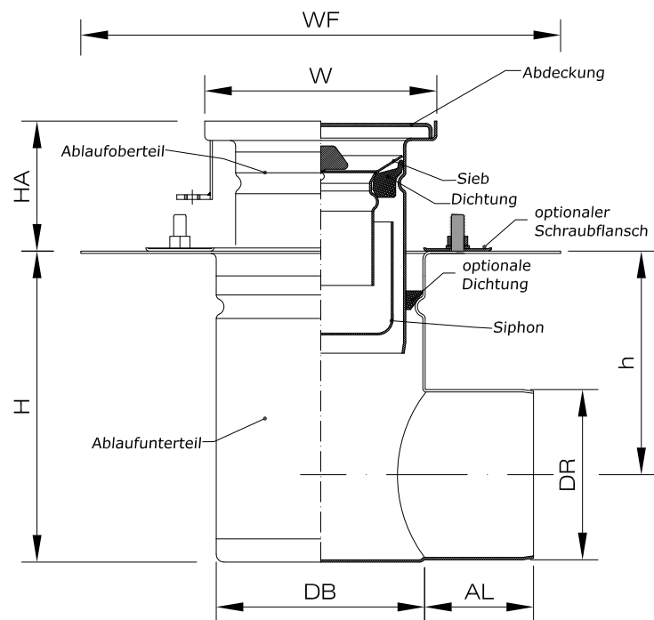
Fliesenklebeflansch, Fliesenabschluss bauseits
