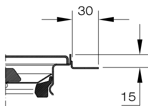
Optional umlaufender Klebeflansch (bei Einbaumaß berücksichtigen !)
